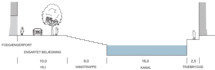
Snit E-E
