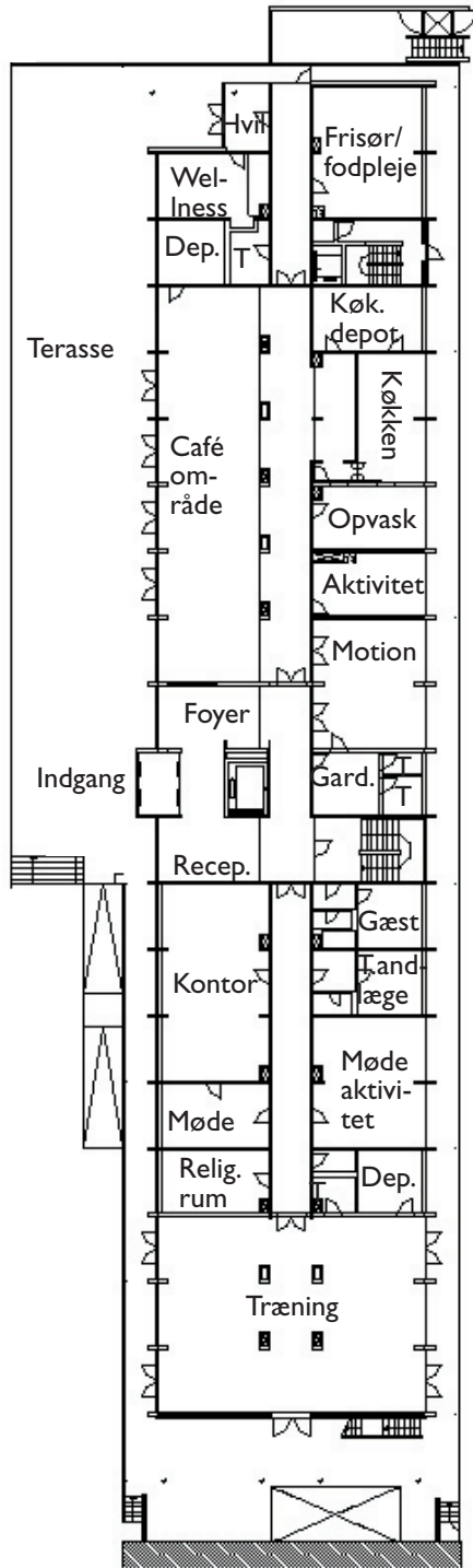
Stueplan
