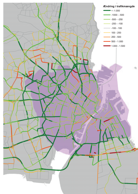
Figur 5.2 Absolut ændring i trafikmængde, døgntakst
