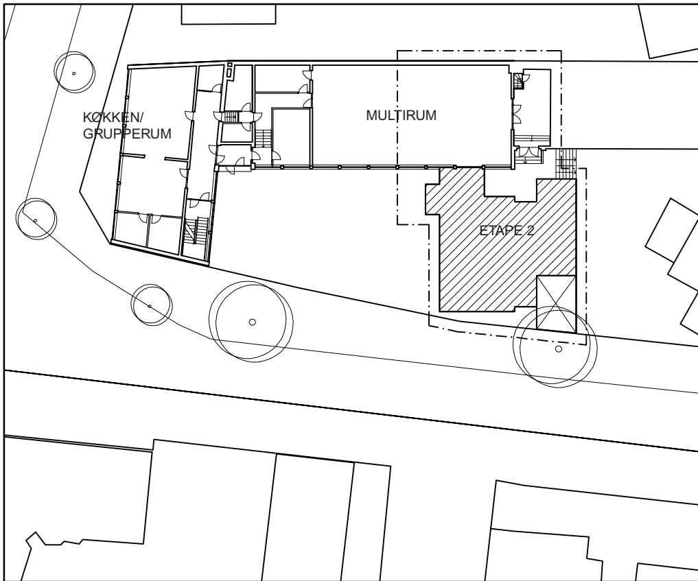
Etape 1 og 2 Situationsplan med stueplan
