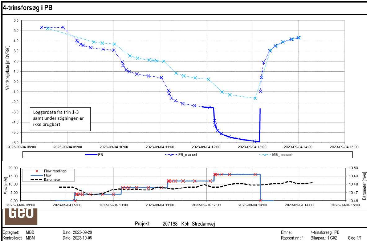
Figur 2 Rådata fra den trinvisse prøvepumpning af PB som optegnet af GEO.
