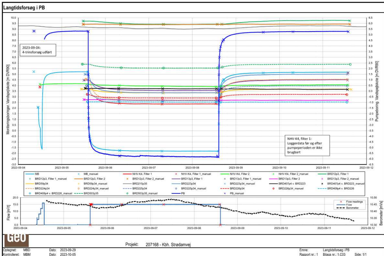
Figur 3 Rådata fra prøvepumpningen med konstant kapacitet som optegnet af GEO.
