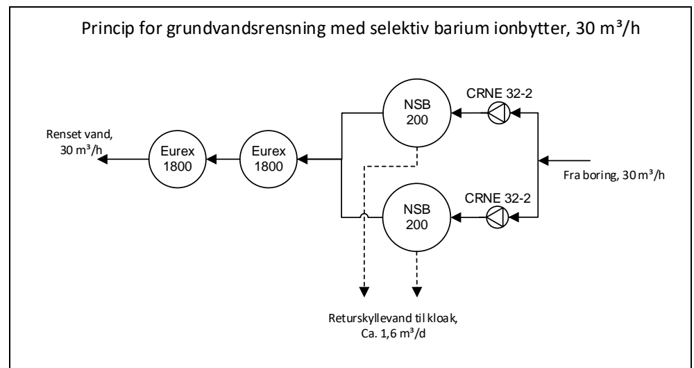
Figur 4-7 Princip for grundvandsrensning med selektiv barium ionbytter ved 30 m 3 /t.
