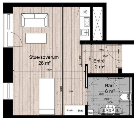
Plan af bolig type B - mellem plejebolig 3 stk. - 36,9 m 2 (netto)
