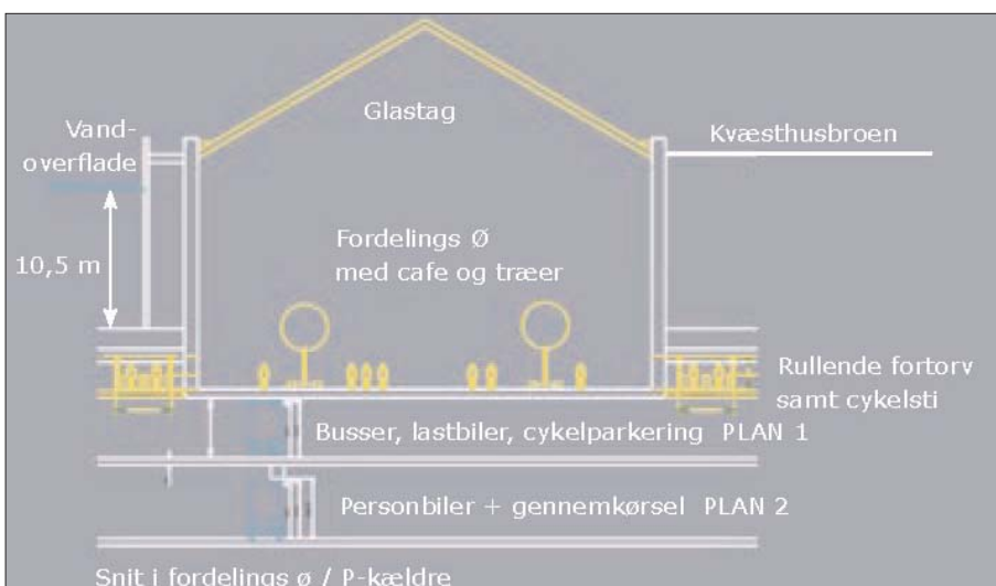
Skitse til City Terminalens glasoverdækkede fordelings ø midt i havneløbet
