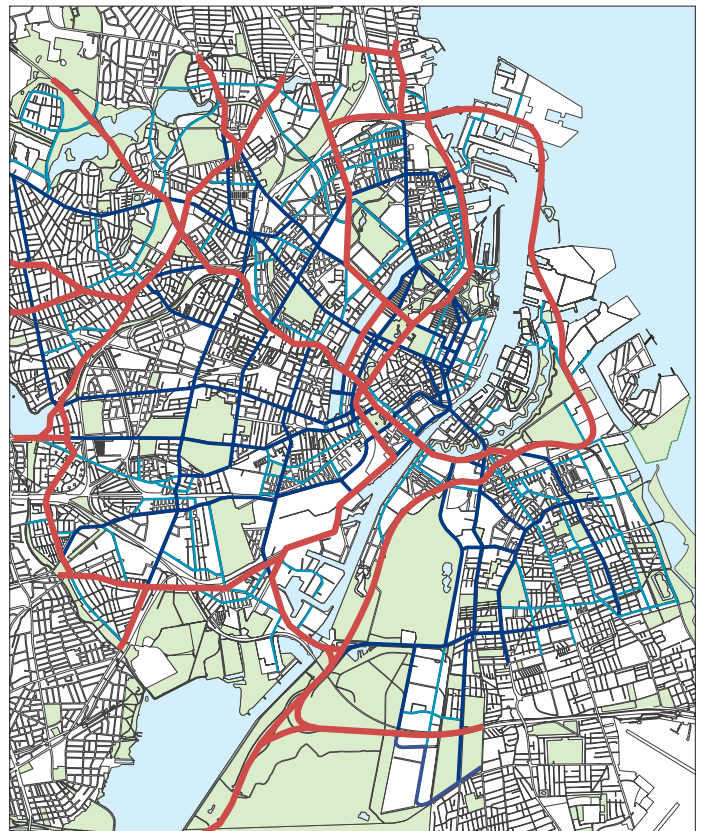
Eksempel på overordnet vejnet med havnetunnelforbindelse over land.
