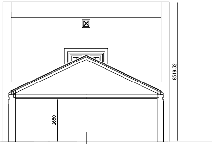
TVÆRSNIT TILBYGNING
