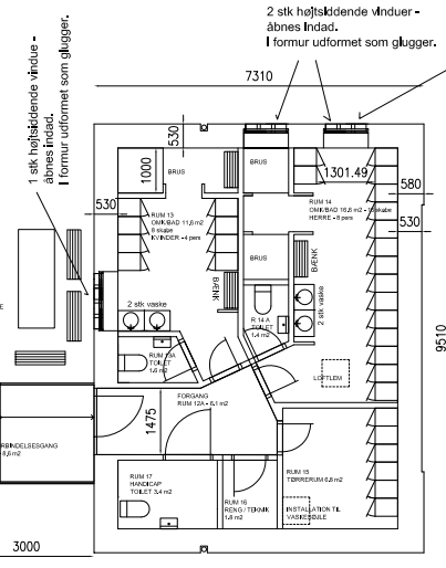
TILBYBYGNING
