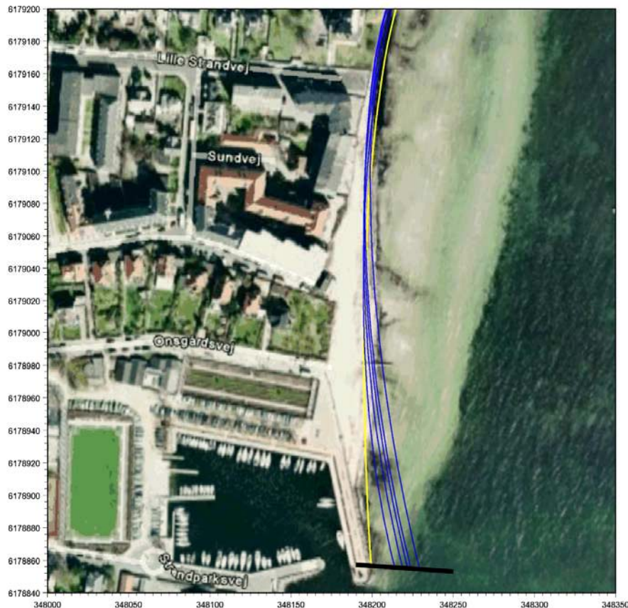
Simulering af strandlinje efter konstruktionen af 50 m lang højde nord for indsejlingen til Hellerup Havn med fremtidigt bølgeklime. Gul kurve: Stabil kystlinje for nuværende forhold. Blå kurver: Fremtidige kystlinjer efter 2, 4, 6, 8 og 20 år. Højde vist med sort signatur.
