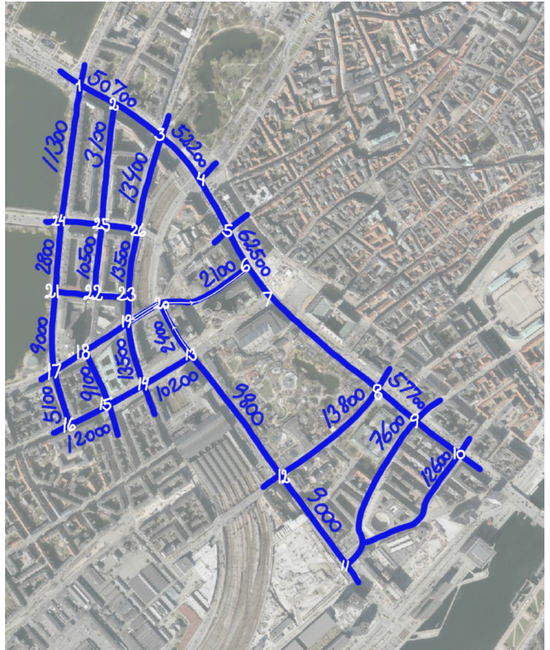
Figur 25. Scenarie 4 - Trafiktal
