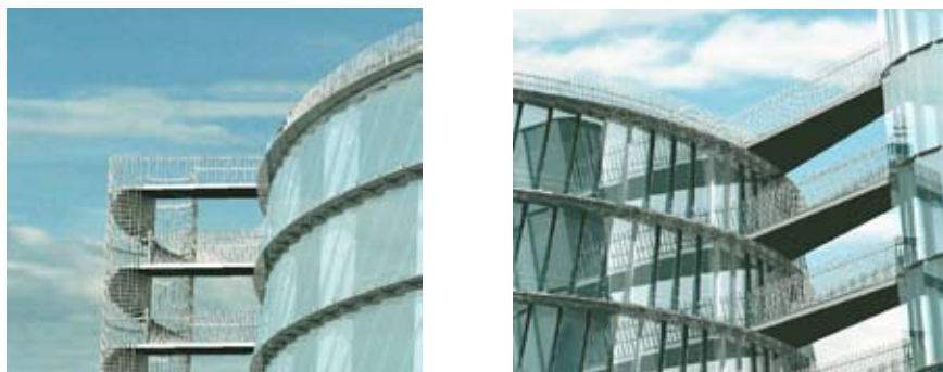
Illustrationerne principiel opbygninger for transparante trappetårne og opbygning af værn.
