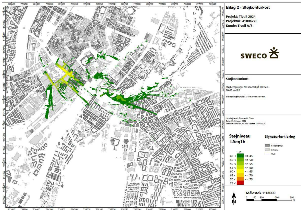
Figur 9-4 Støjdbredelse 1,5 m over terrænen ved afholdelse af koncerter på Plænen med grænseværdi 60 dB(A)
