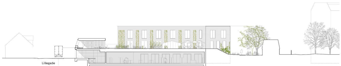
Principalsnit BB, der viser et eksempel på et nybyggeri i sammenhæng med omgivende eksisterende bygninger i overensstemmelse med lokalplanen. Illustration: Entasis.
