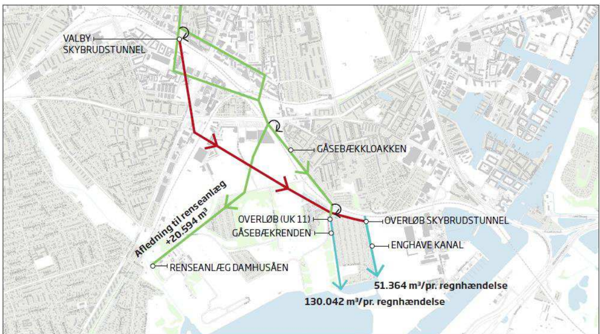
Figur 4.3 Hovedforslag. Udlledning til Gåsebækkrenden og Enghave kanal ved kraftigt skybrud/100 års-hændelse (eksemplificeret ved nedbørshændelsen 2. juli 2011) i dag (øverst) og fremtidigt med Valby Skybrudstunnel (nederst) for en løsning med overløbskant.
