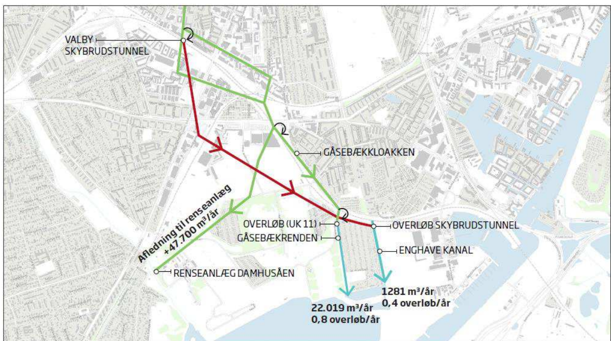
Figur 4.1 Hovedforslag. Udlledning til Gåsebækrenden og Enghave kanal ved hverdagsregn i dag (øverst) og fremtidigt med Valby Skybrudstunnel (nederst) for en løsning med overløbskant.
