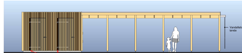
④ Halvtag - Vest 1:50
