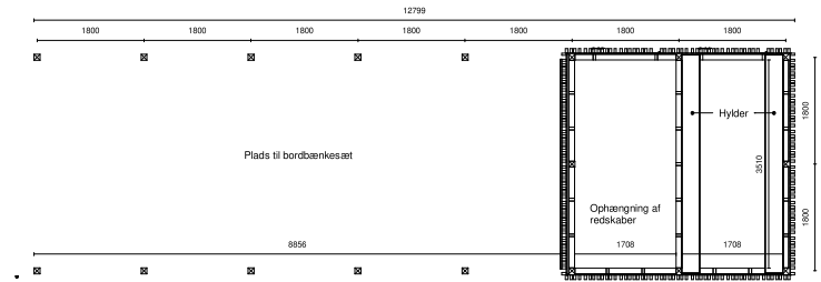
⑤ Halvtag - Nord 1:50
