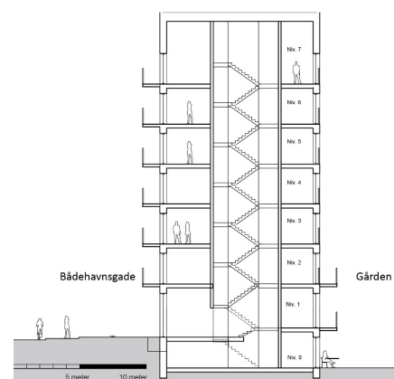
Snit, der viser håndtering af terrænspring i boligerne langs Bådehavnsghade i overensstemmelse med lokalplanen. Illustration: DesignGroup Architects.
