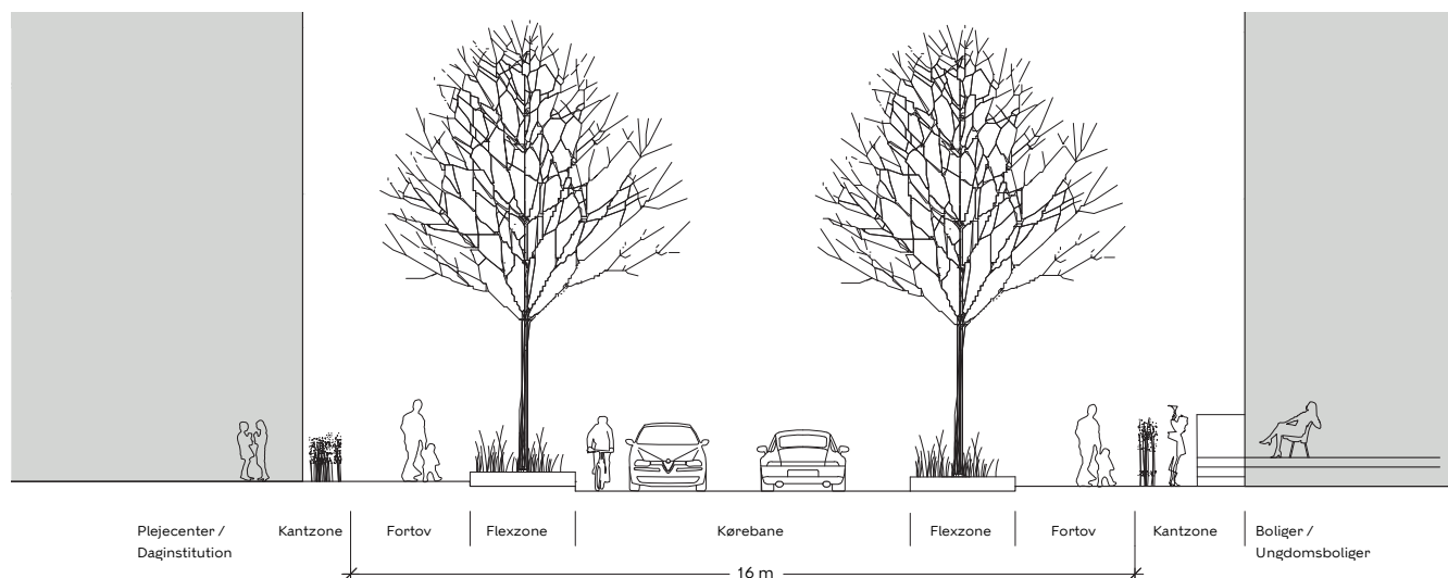
Snit A-A
