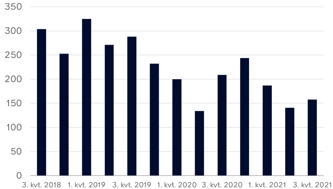
Figur 3. Antal formalitetssklager
