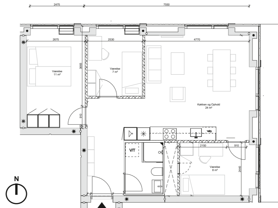
Boligplan
