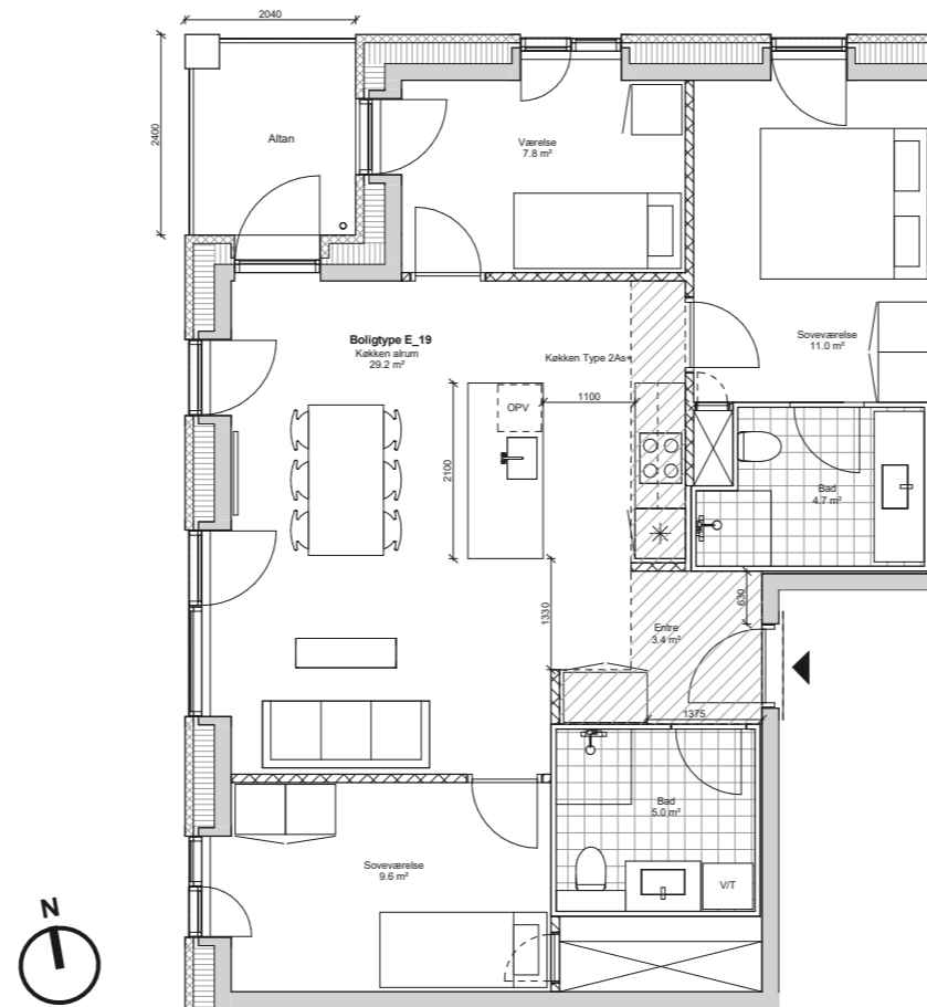
Boligplan
