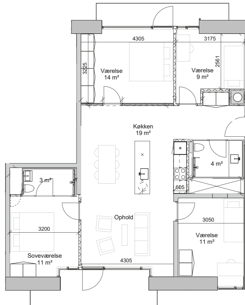
Boligplan
