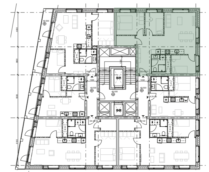
Etageplan
