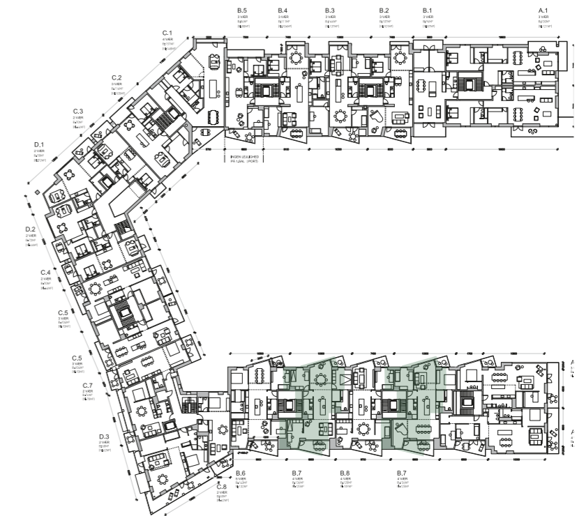
Etageplan
