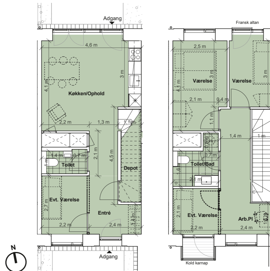
Boligplan
