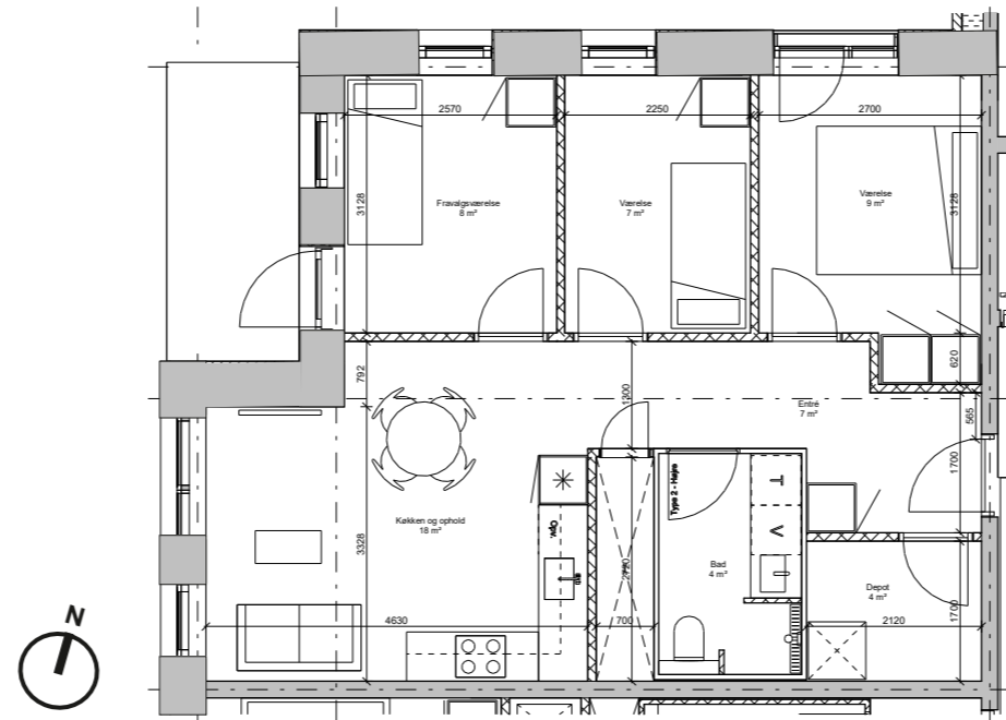
Boligplan
