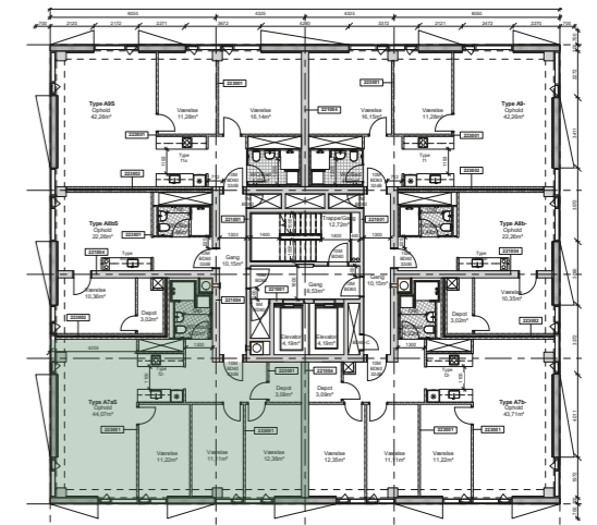
Etageplan
